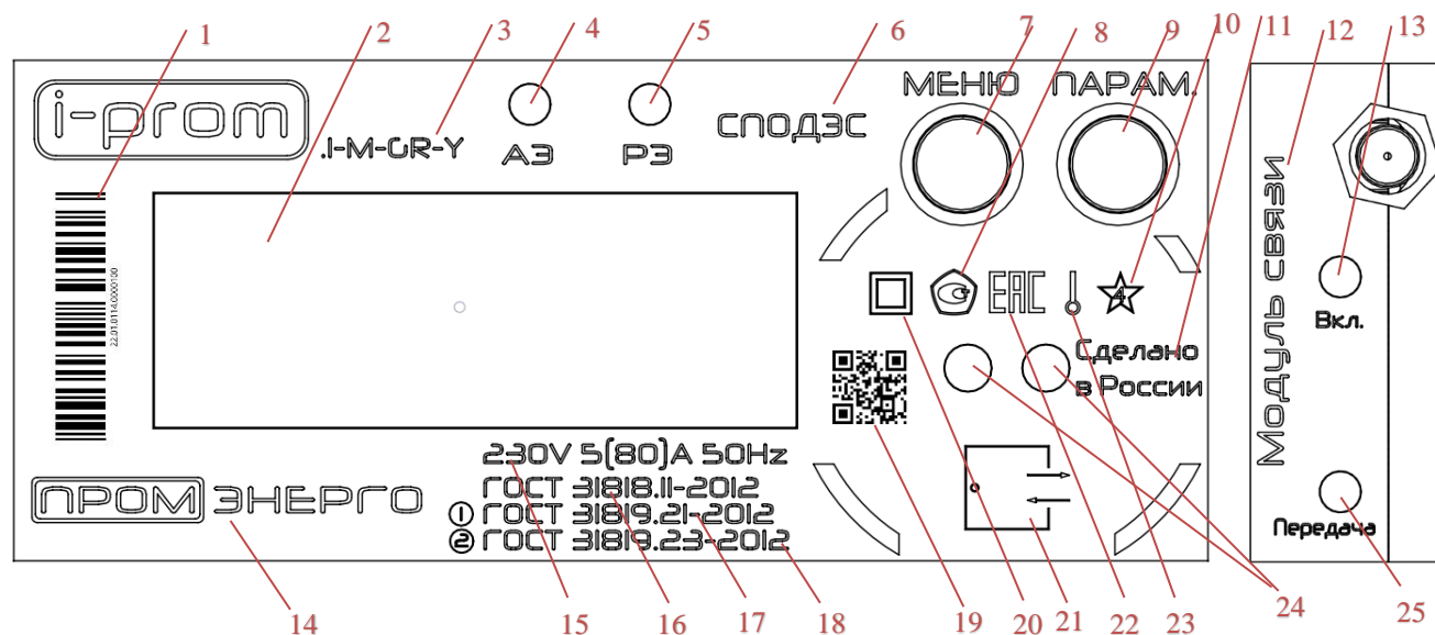
Рисунок 4.2 - Маркировка счётчиков электрической энергии однофазных многофункциональных i-prom.1
