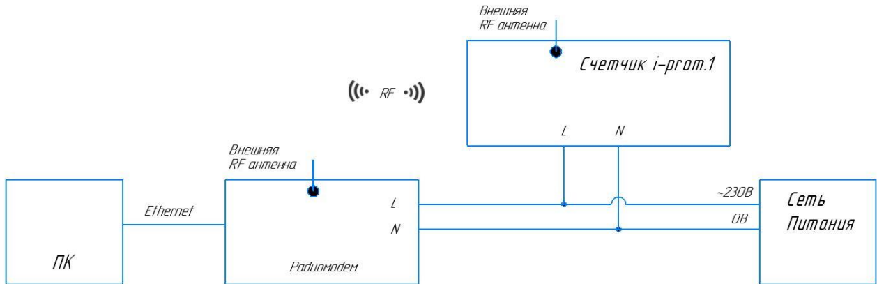
Рисунок В.7 – Схема подключения счетчика к ПК через интерфейс GSM
